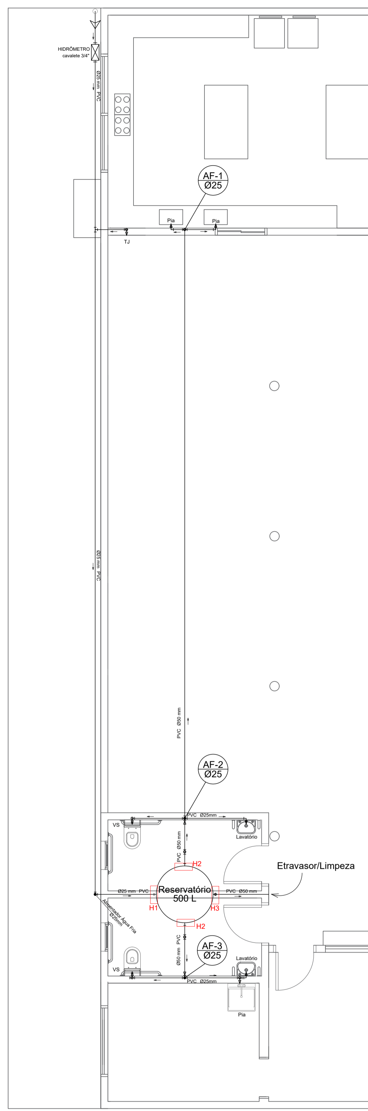
Planta baixa Hidráulica Escala 1:50
