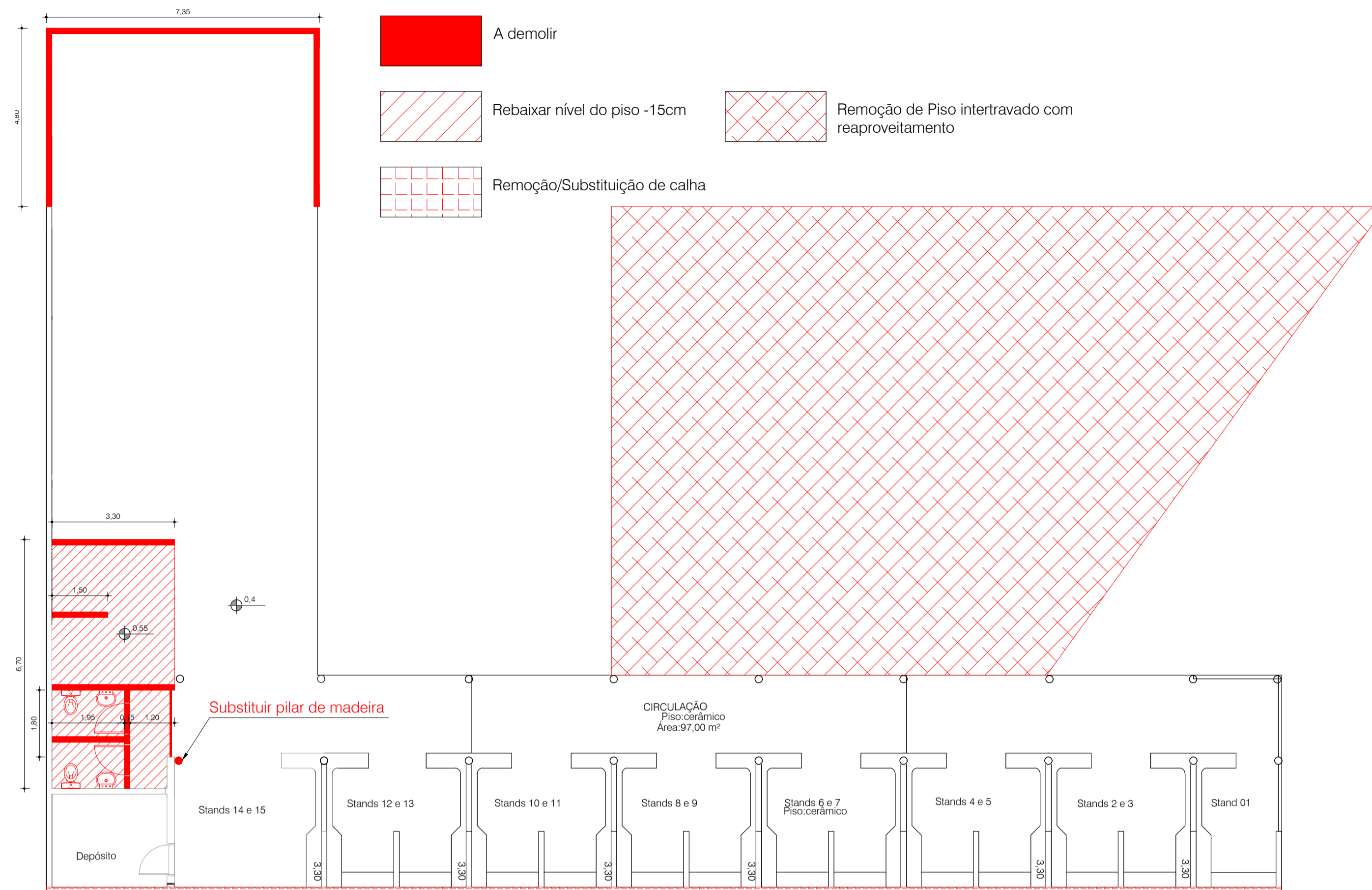
Planta de demolição Escala 1:100
